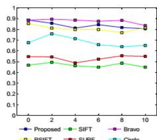
(d) JPEG-Compression
