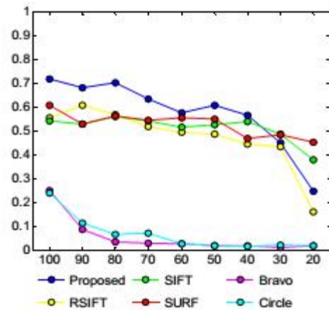
(d) JPEG-Compression
